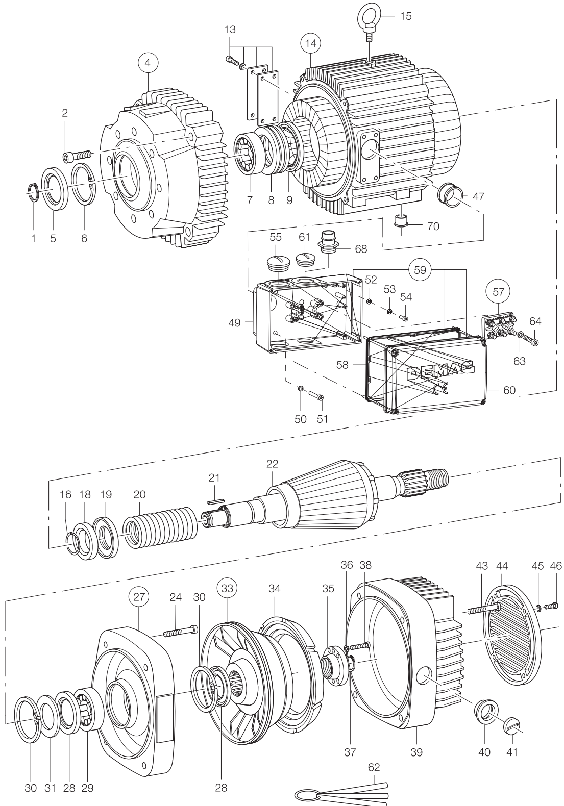
Motor KBH 225 B6
